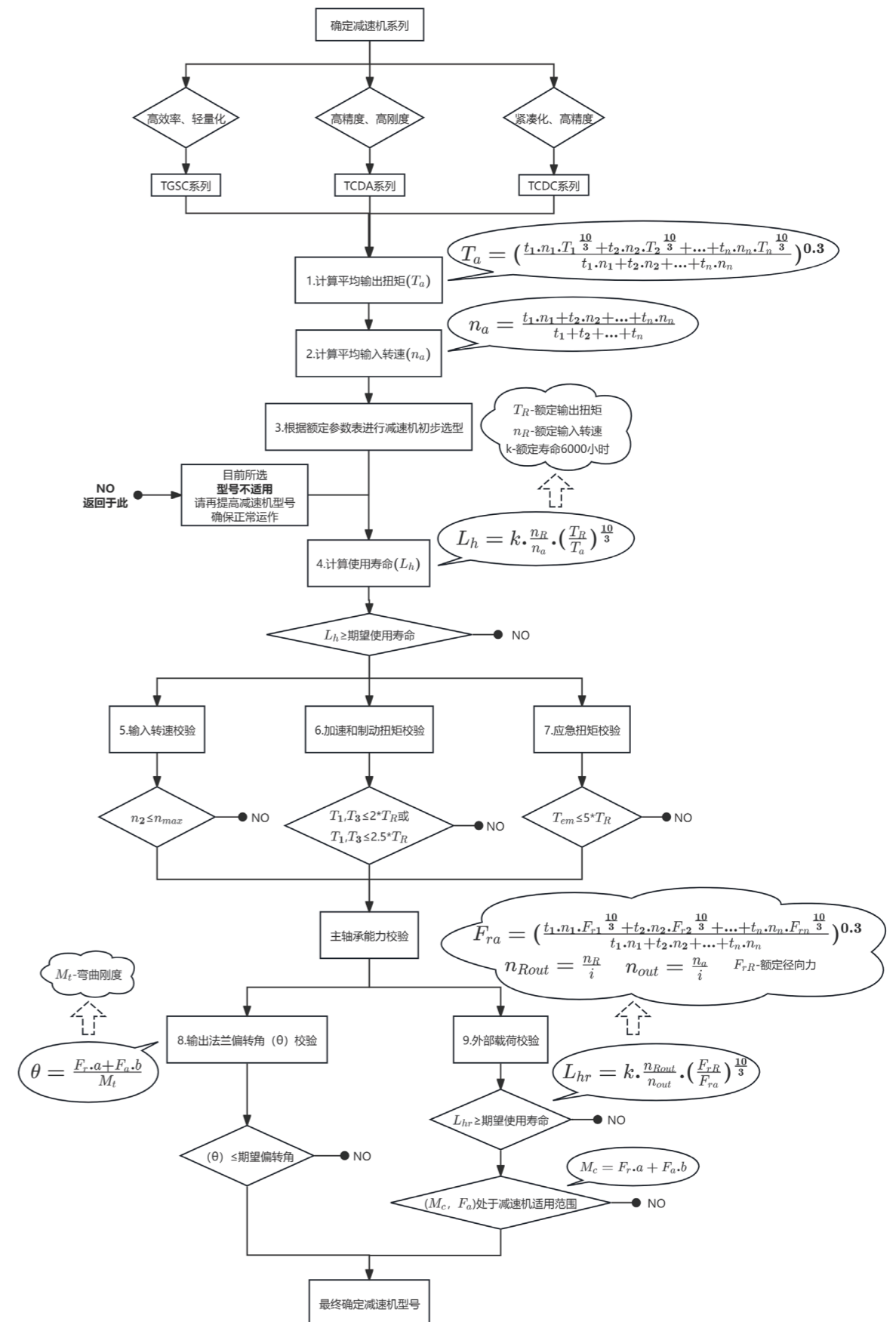
TGSC, TCDA, TCDC系列选型流程
